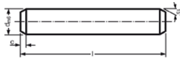
ISO 2338
